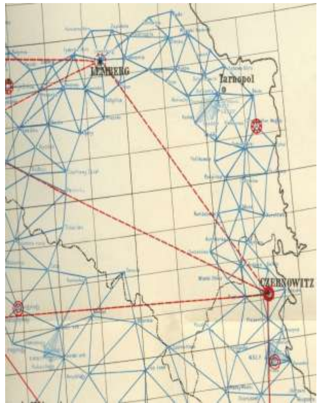
Рис.2 Мережа тріангуляції 1-го класу, геодезичні бази та астрономічні пункти, закладені на яких проведено спостереження Віденським ВГІ.
